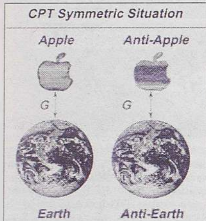
Zemlja privlači jabuku, antizemlja privlači antijabuku
