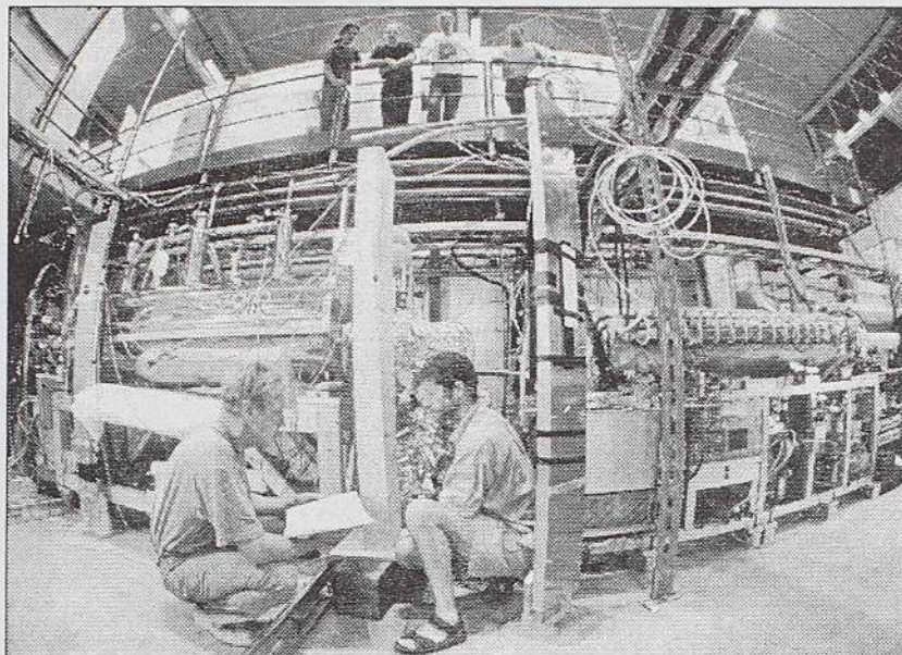
Fotografija složene aparature ATHENA koja proizvodi antivodonikove atome
