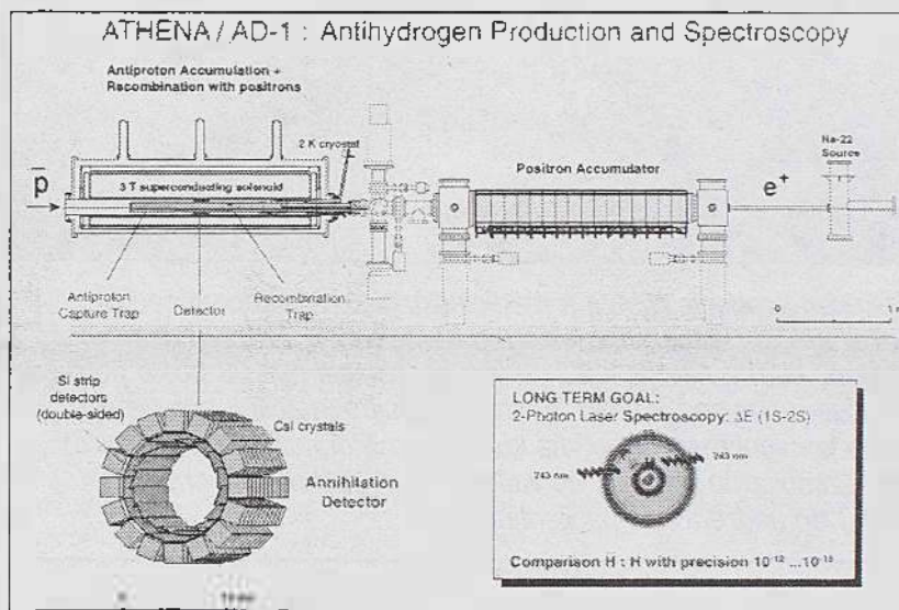
Schematski prikaz nastajanja antivodonika u ATHENI
